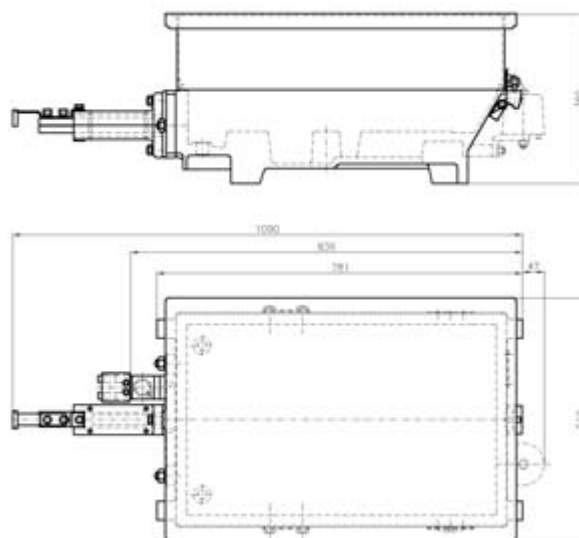
Schéma skříně přestavníku
